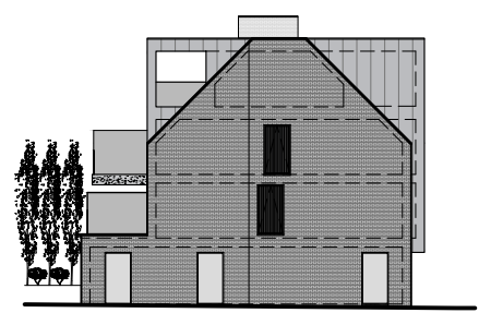
LINKERZIJGEVEL OVERZICHTSPAN VERDIEPING +2
